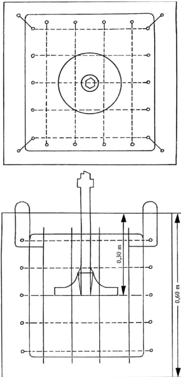
Figura 10.2 Bloc d'assaig
