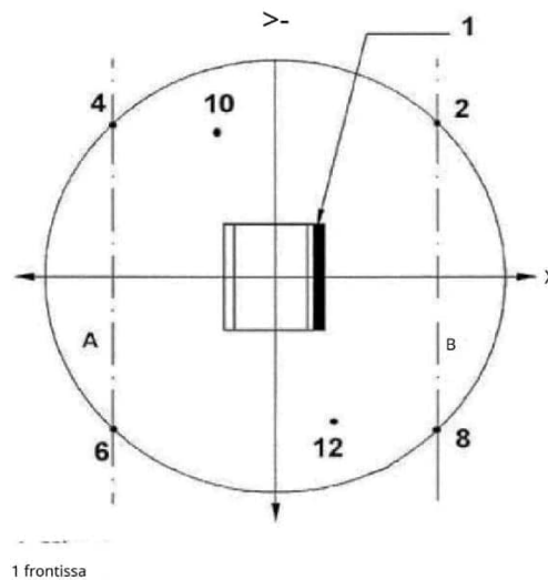
Figura 39.3 Distància de mesurament
