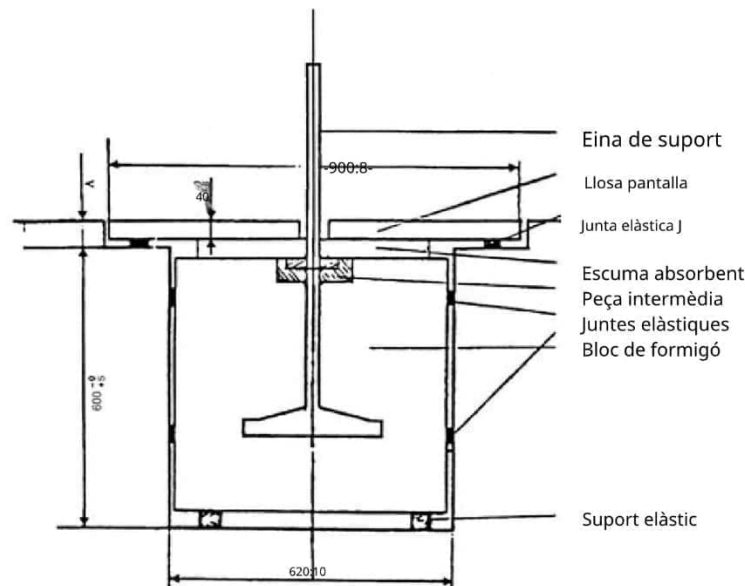
Figura 10.3 Dispositiu d'assaig
