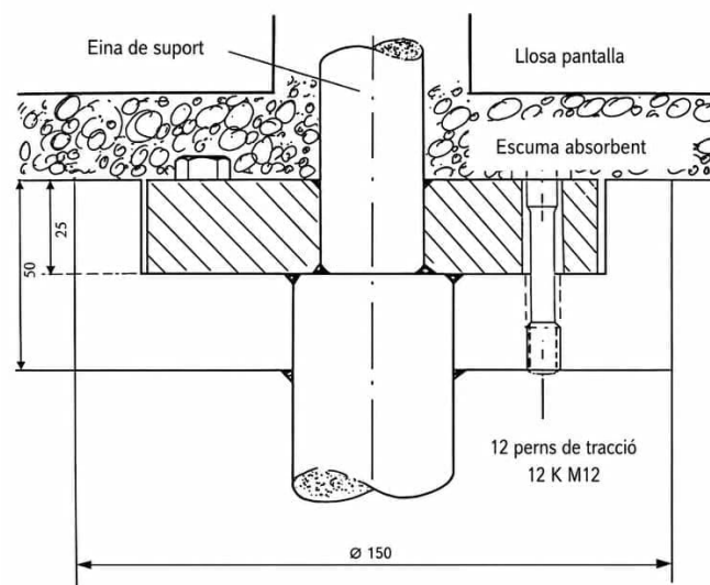
Figura 10.1 Esquema de la peça intermèdia
