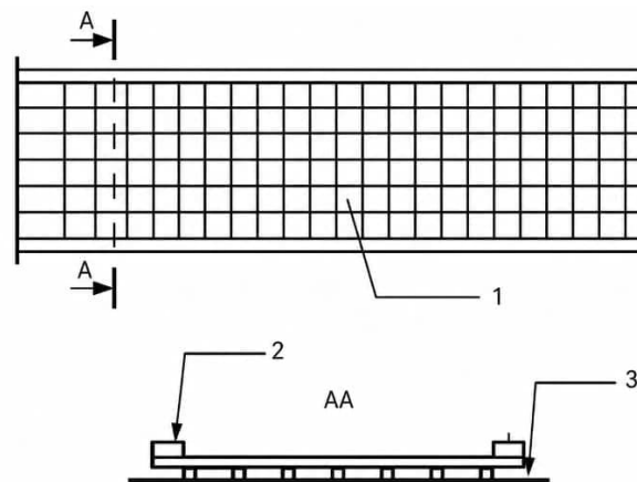
Figura 39.2 Detall de la construcció i muntatge de la pista de rodament
