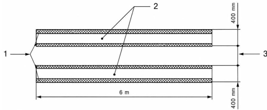
Figura 39.1 Dibuix de la pista de rodament
