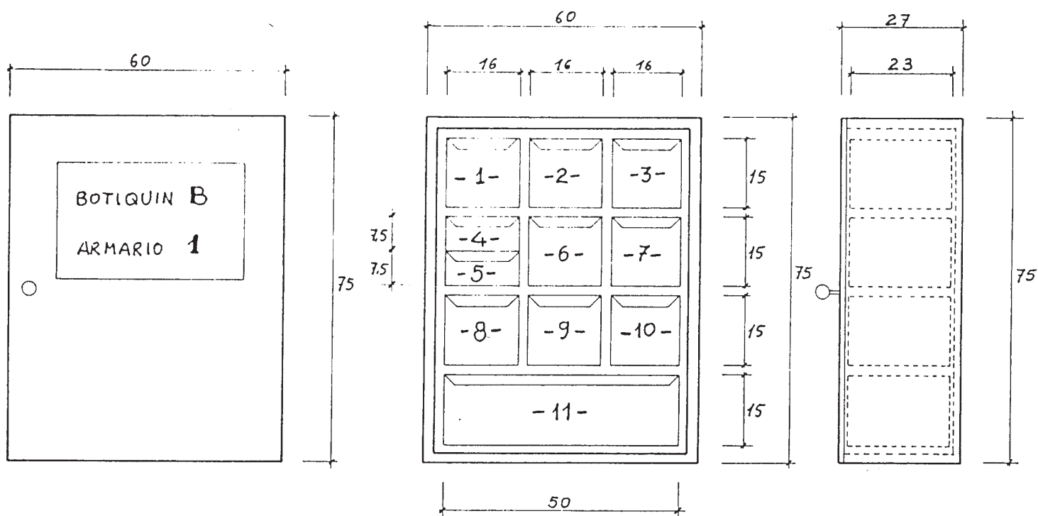
VISTA FRONTAL (CERRADO)
