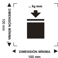
Embalajes/envases de gran tamaño apilables
