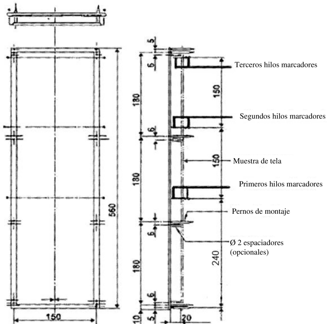
Figura 1 Portamuestras (dimensiones en milímetros)
