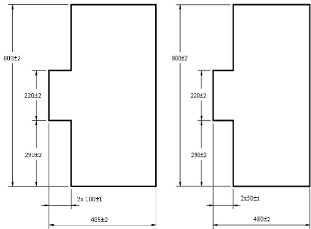
Figura 3 Dimensiones del material de recubrimiento (dimensiones en mm)
