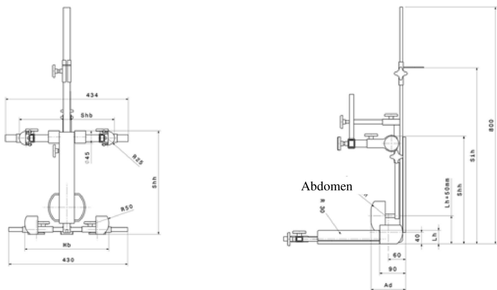
Vista lateral y frontal del dispositivo de medición para mediciones aplicables a sistemas reforzados de retención infantil con pantalla anticoliisión
