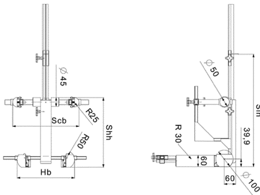
Dispositivo de medición del SRIR. Vista lateral y frontal del dispositivo de medición
