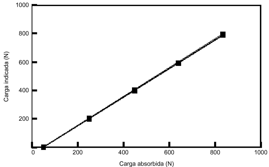
Carga indicada a 80 km/h en función de la carga absorbida a 80 km/h
