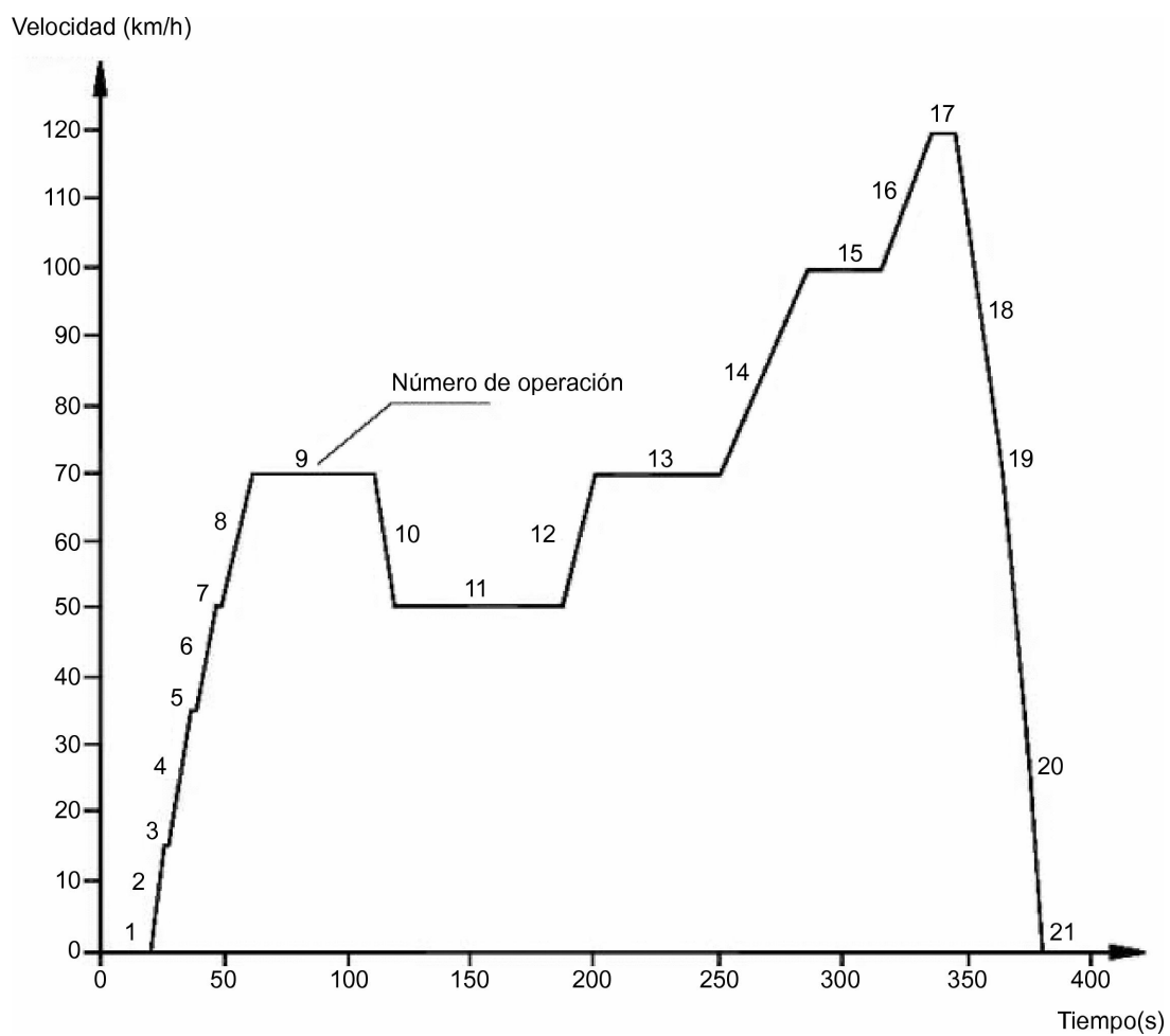
Figura 1/3 Ciclo extraurbano (parte 2) del ensayo del tipo I
