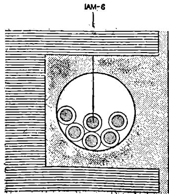
Sección
