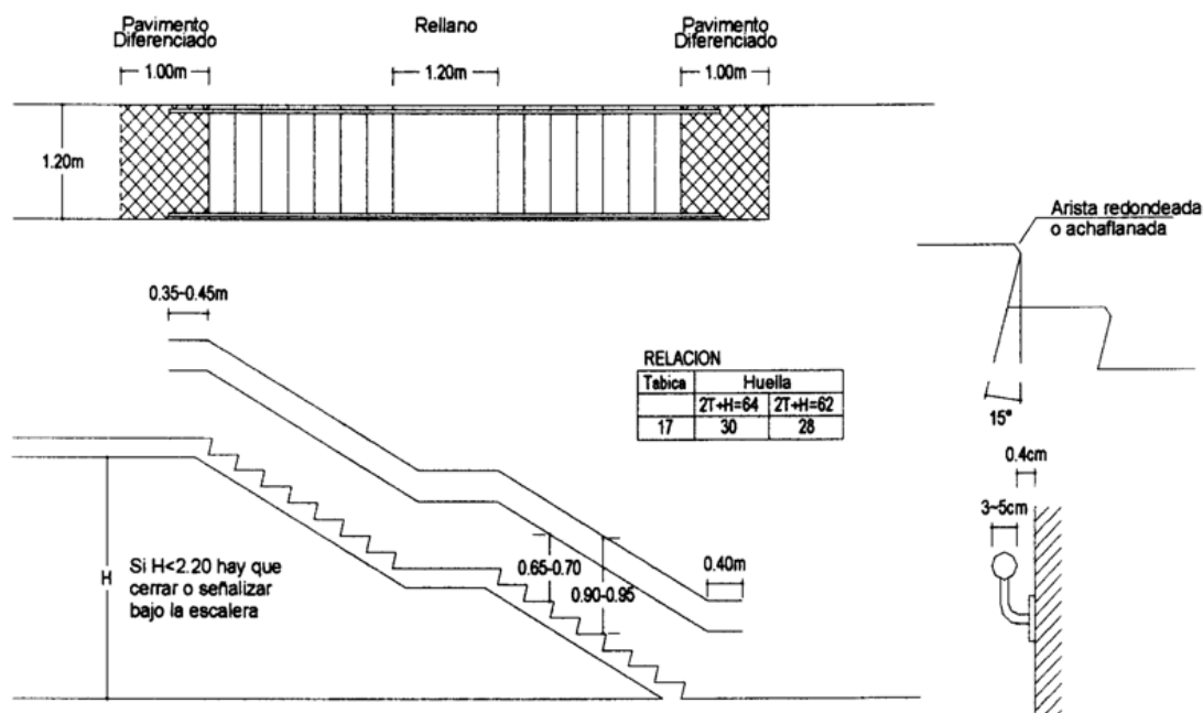
FIG. 1.2.3 ESCALERAS
