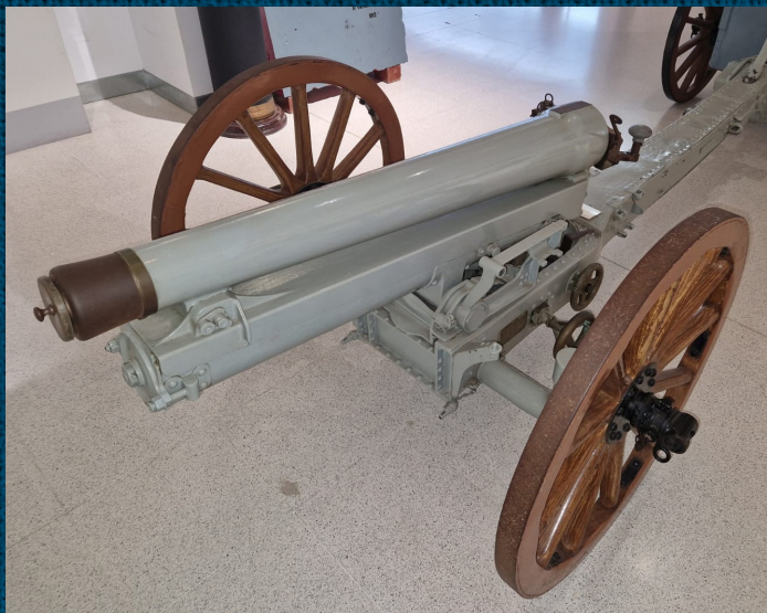
Cañón Vickers de desembarco de 76,2 mm/17 del acorazado Jaime I que fue agregado a las tropas de tierra para aumentar la potencia de fuego de la artillería de campaña (© Museo Naval de Cartagena)
