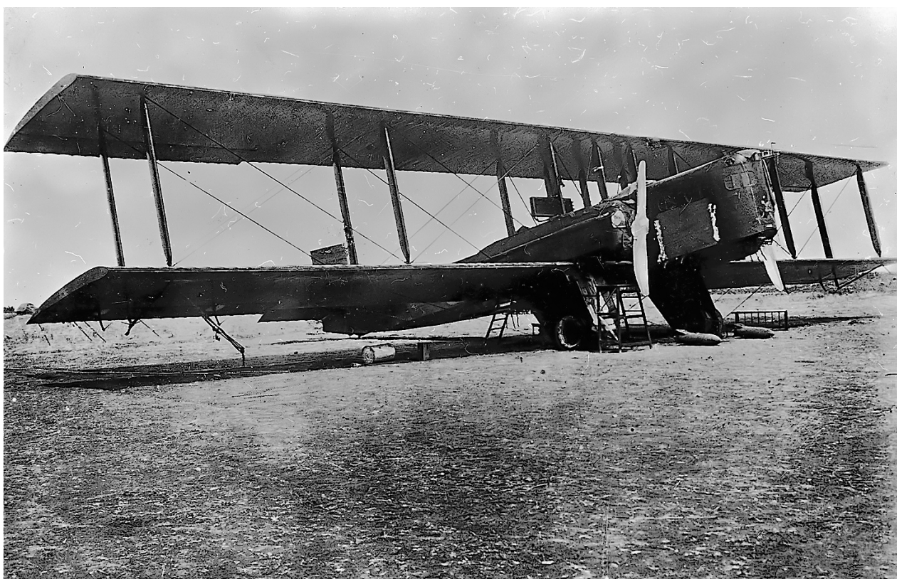
Bimotor Farman Goliath F-60 . Motores Lorraine 12D, de 375 CV. (4,5 x 6 cm a 9 x 12 cm) (AHEA. Centro Cartográfico y Fotográfico. Signatura procedencia: 11923-1.º A.C. Serie 2.º. Número Cartera [Ob]: 1139 Negativo [Ob]: 01)
