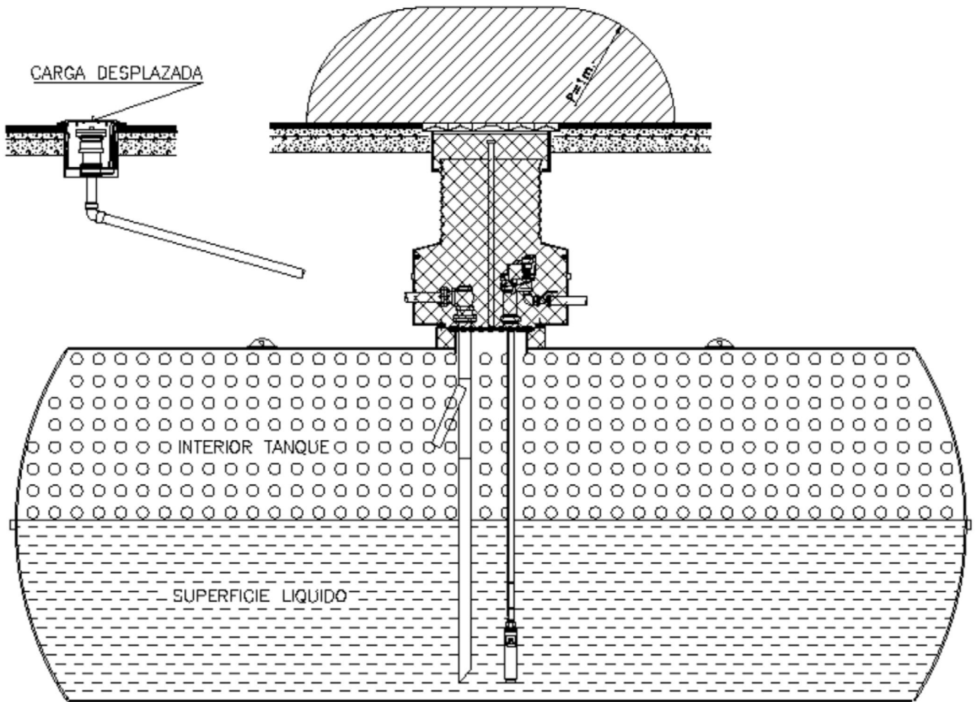
Figura 3. Detalle de clasificación de zonas de arqueta boca de hombre sin puntos de escape
