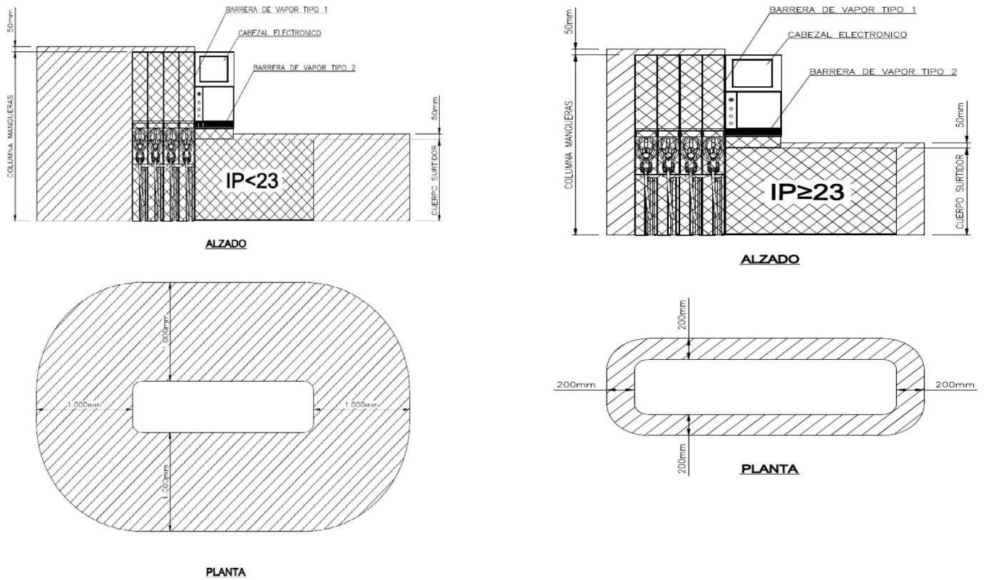
Figura 1. Detalles de clasificación de zonas de surtidores según el grado de protección de la envolvente
