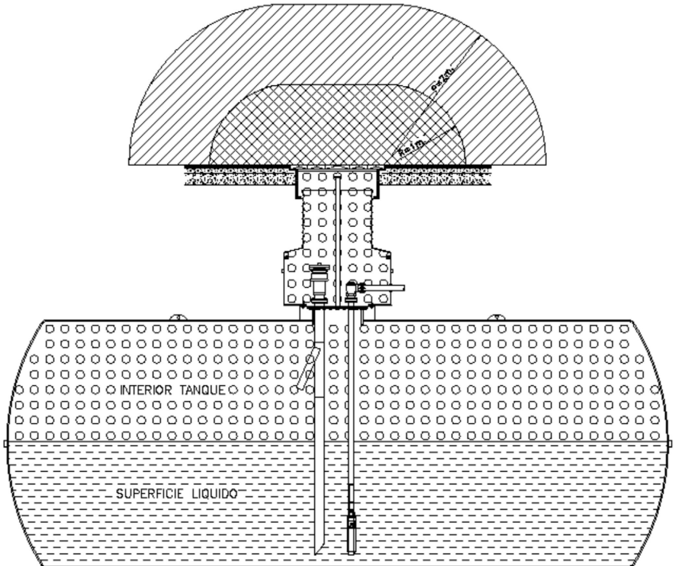
Figura 2. Detalle de clasificación de zonas de arqueta boca de hombre con fuentes de escape
