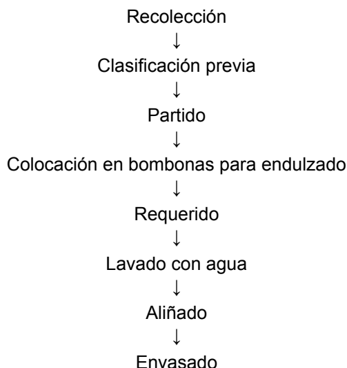
Figura 5.1 Esquema de elaboración de aceitunas verdes frescas.
