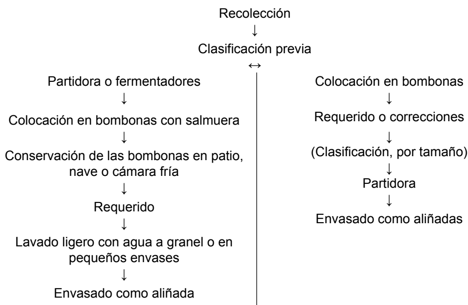
Figura 5.2 Proceso de elaboración de las aceitunas fermentadas.
