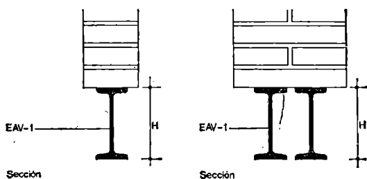
Sección
