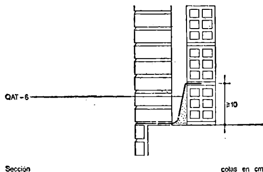
Sección
