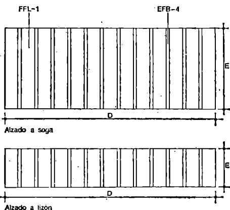
Alzado a tizón
