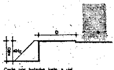
Corte por batache junto a vial
