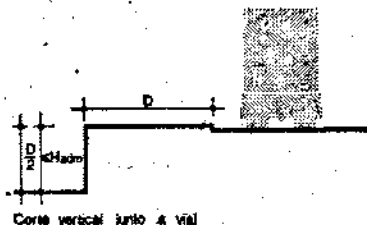
Corte vertical junto a vial
