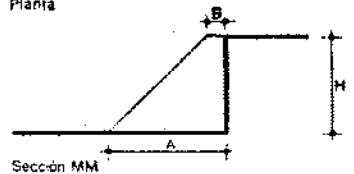
Sección MM'
