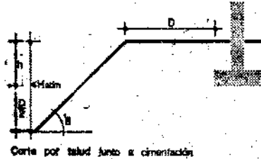
Corte por talud junto a cimentación
