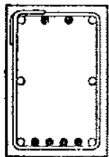
○ Armadura de torsión A_s TOR ● Armadura de flexión A_s, A_s'
